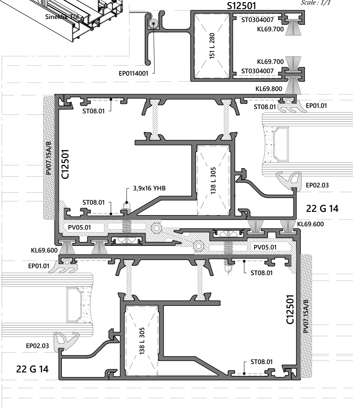
ÖLÇEK : 1/1 Scale : 1/1
