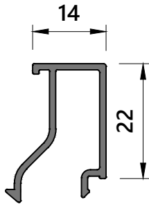
22 G 14 Cam Çıta Pr. 0,233 kg/m
