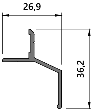
P12501 Damlalık Prof. 0,248 kg/m
