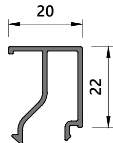
22 G 20 Cam Çıta Pr. 0,253 kg/m
