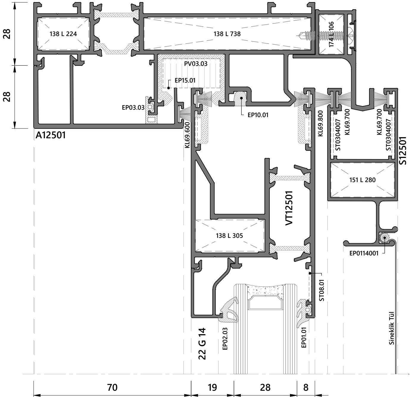
ÖLÇEK : 1/1 Scale : 1/1
