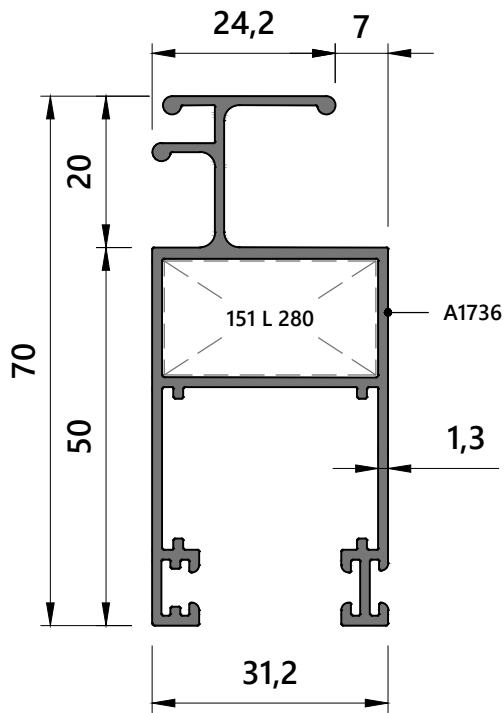
S12501 Sin.Kanat Pr. 0,884 kg/m
