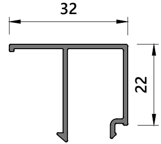
22 G 32 Cam Çıta Pr. 0,284 kg/m
